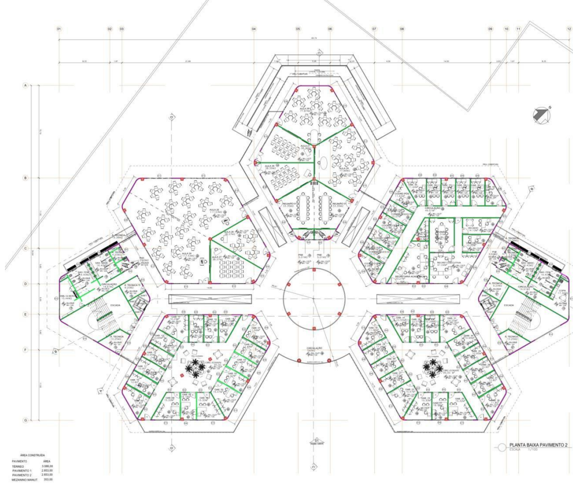
Figura 9: Planta do Segundo Andar do Núcleo Pedagógico
