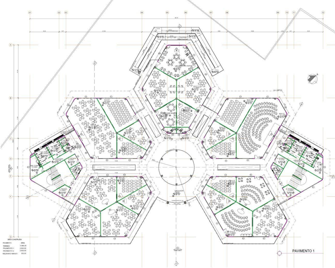
Figura 8: Planta do Primeiro Andar do Núcleo Pedagógico
