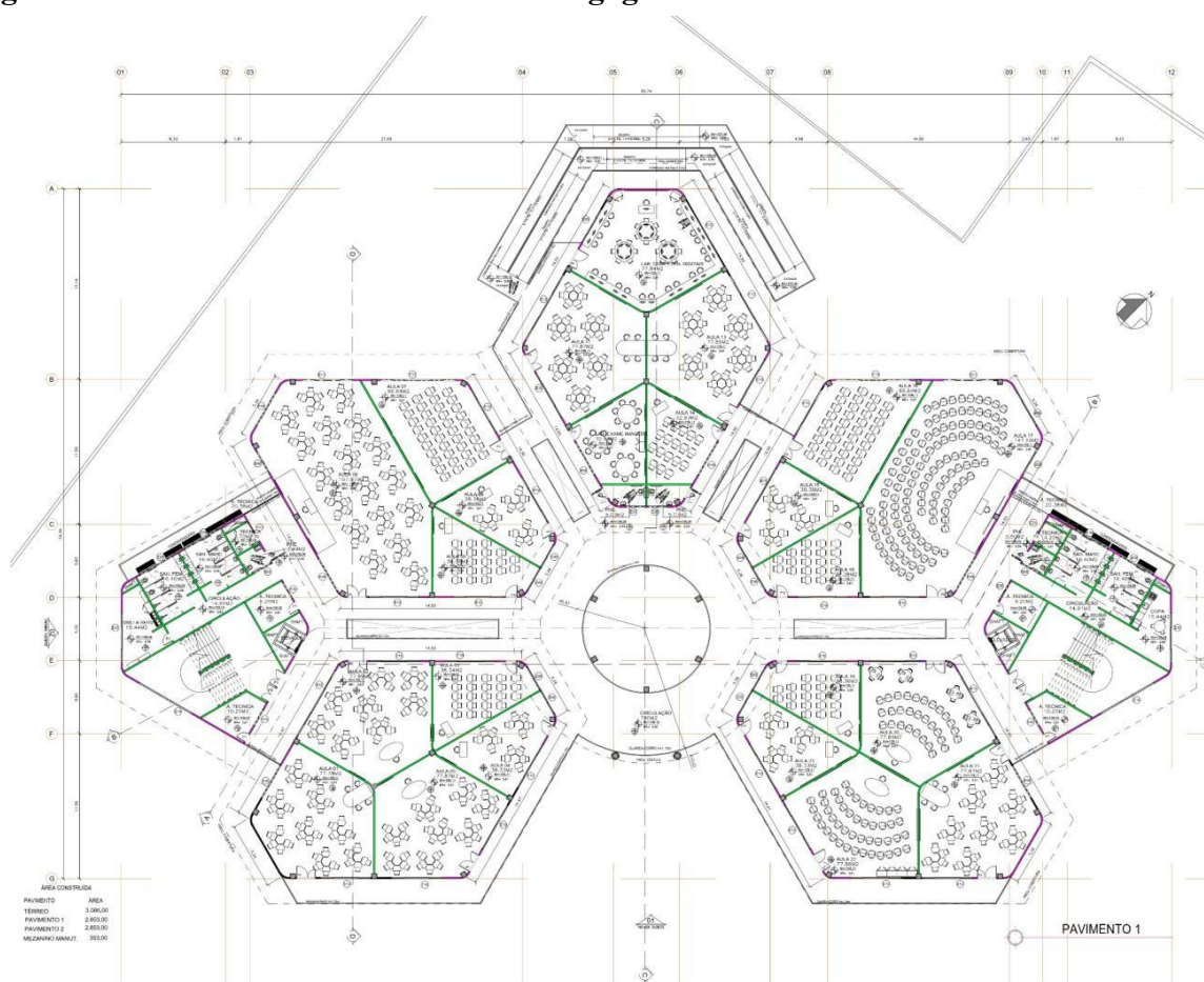
Figura 7: Planta do Térreo do Núcleo Pedagógico
